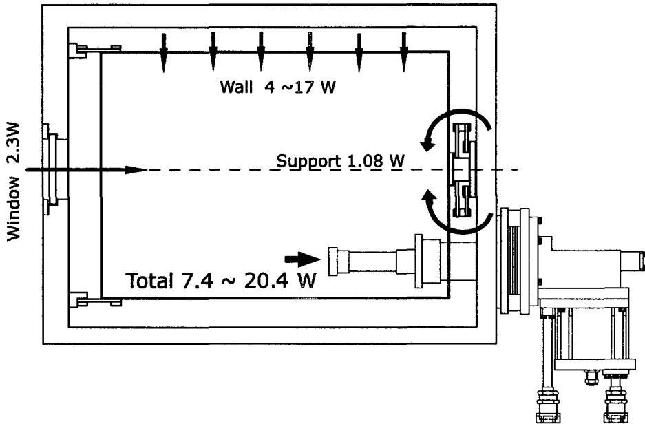
그림 5. Cold-Box 열 유입량(단면도).
