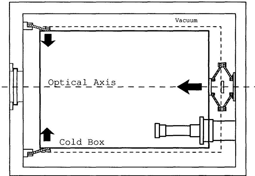
그림 4. Cold-Box 지지 방법(단면도). 점선은 상온에서의 Cold-Box 수축 전 모습, 굵은 실선은 수축 후 모습. Cold-box를 지지하고 있는 Fiberglass로부터의 열 유입량을 고려하였음.
