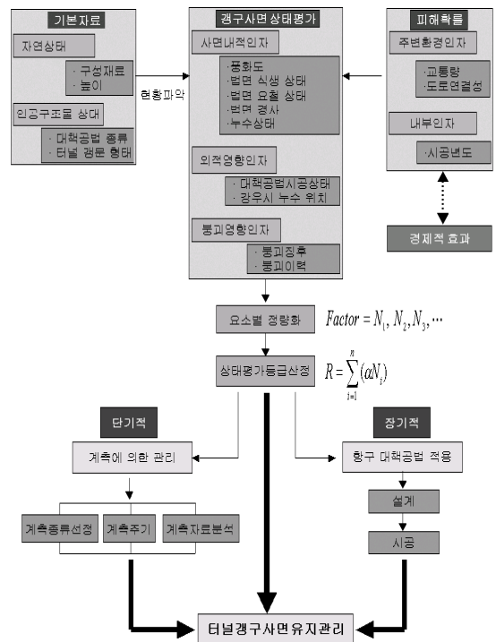
그림 5. 터널 갱구사면 상태평가 흐름도
