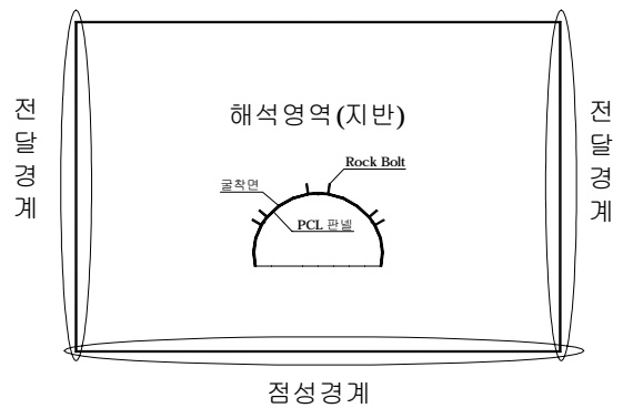
그림 8. 해석모델의 경계조건
