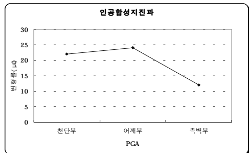
그림 5. 진동대실험으로 부터 얻어진 PCL의 최대변형률
