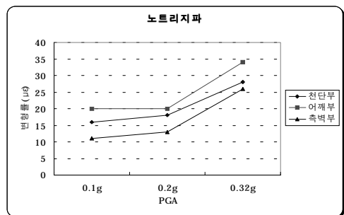
(b) 노트리지진파
