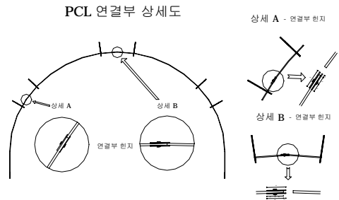
그림 3. 모형 PCL의 상하부패널 연결방식
