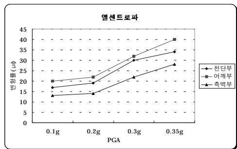
(a) 엘센트로지진파
