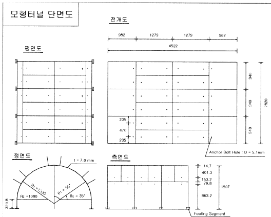
그림 2. 진동대 실험용 PCL모형체
