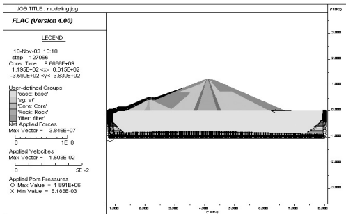
그림 4. 해석 모델링
