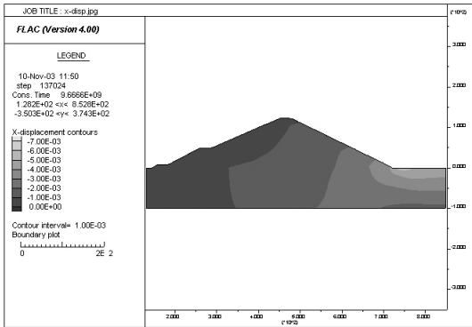
그림 14. 수평 변위도
