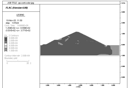
그림 21. 간극수압 분포도(하중재하 후)
