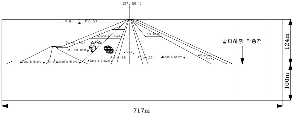
그림 3. 해석 단면도
