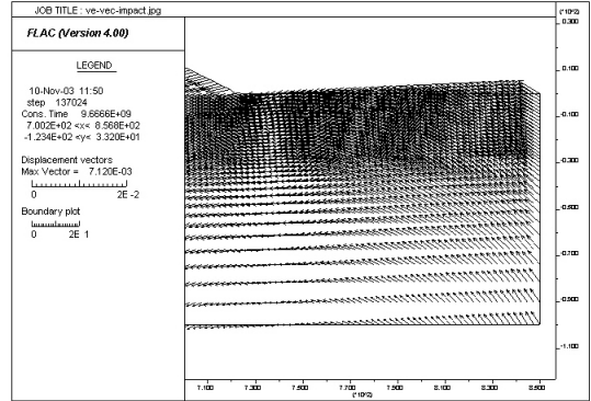
그림 13. 가진점 주위의 변위 벡터도
