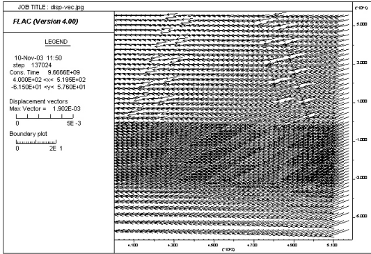
그림 12. 코어 중심부의 변위 벡터도
