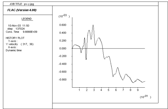
그림 7. 코어 중심부의 수직방향 입자속도
