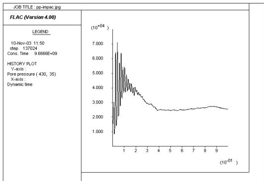
그림 16. 가진점의 과잉간극수압 발생경향 (1초)
