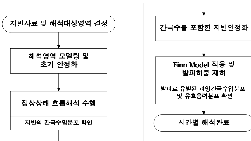
그림 1. 검토흐름도
