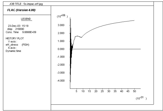
그림 19. 가진점의 유효응력 변화경향 (5초)
