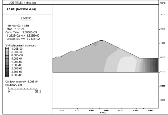
그림 15. 수직 변위도
