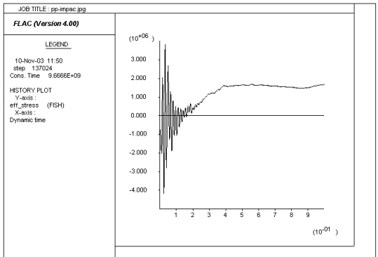
그림 17. 가진점의 유효응력 변화경향 (1초)
