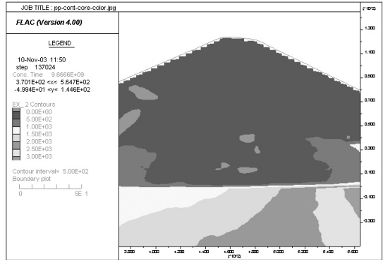
그림 23. 코어 중심부의 과잉간극수압 분포도
