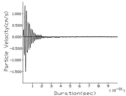
그림 5. 입력하중
