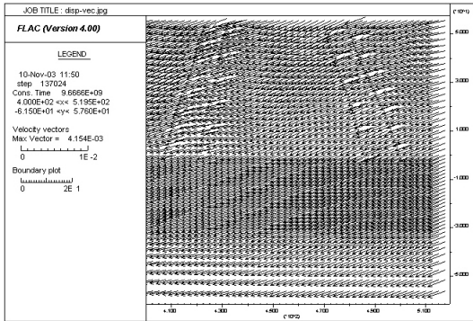
그림 8. 코어 중심부의 속도 벡터도
