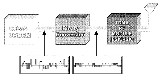
[그림 2] Binary CDMA 개념도
