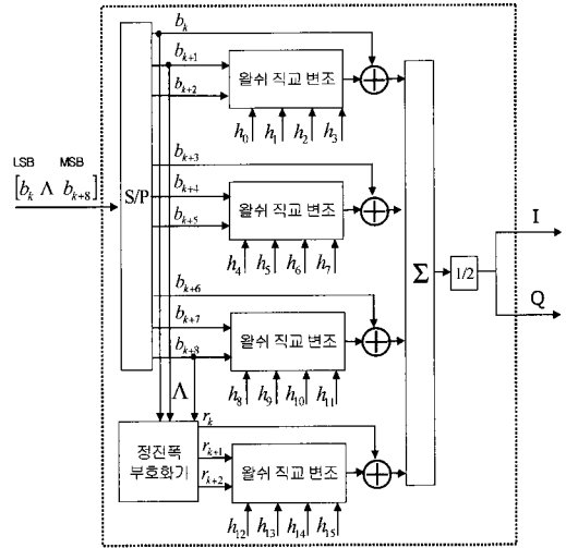
[그림 7] RATE 3의 블럭도
