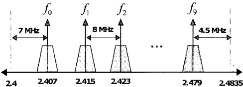
[그림 3] 주파수 대역
