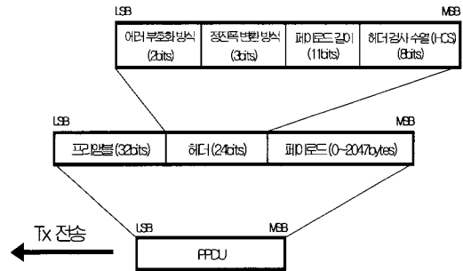
[그림 4] 물리 계층 패킷 형식
