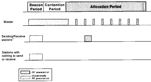
[그림 23] Koinonia 시스템의 기기별 duty cycle
