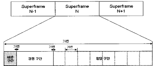
[그림 13] 슈퍼프레임 구조
