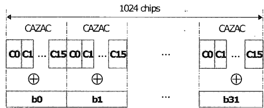
[그림 9] 프리앰블 수열의 구조
