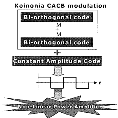
[그림 17] 선형 앰프의 불필요성
