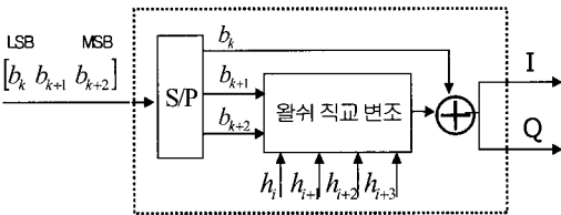
[그림 6] RATE 2의 블럭도
