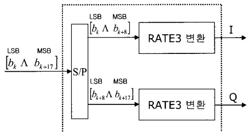
[그림 8] RATE 4의 블럭도
