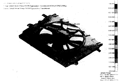
Fig. 7 2 nd mode of CFA : 80 Hz
