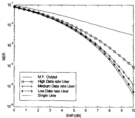
그림 2. K = 9 인 경우 제안된 수신기의 비트 오류율
