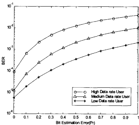
그림 4. E_b/N_0 = 10\text{dB} , G = 3 인 경우 가우시안 환경하에서 비트추정에러 확률에 따른 오류율
