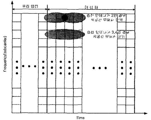
그림 4. OFDM시스템의 프레임 구조
