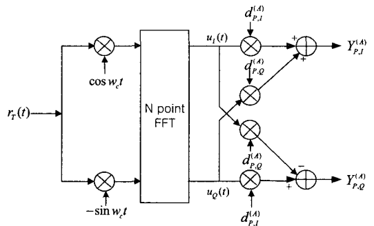
그림 2. 채널 추정을 위한 블록 다이어그램
