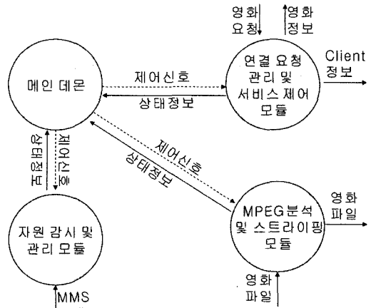
그림 2 HS의 모듈 구성
