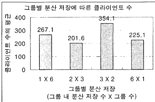
그림 7 그룹별 분산 저장에 따른 성능 측정 결과
