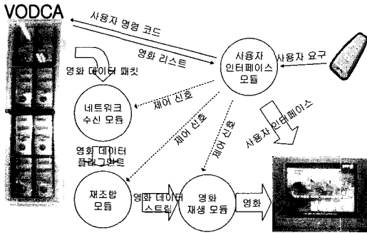
그림 4 내장형 클라이언트의 구성
