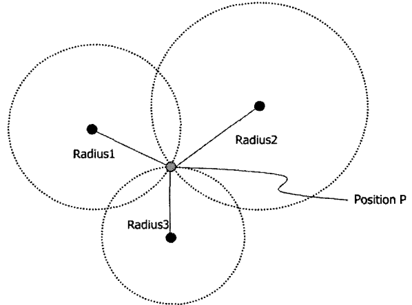
그림 2 ToA 방식
