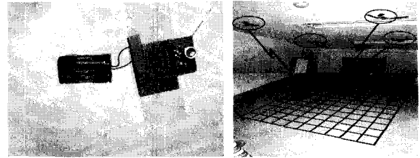
그림 10 천장에 부착된 비컨의 모습
