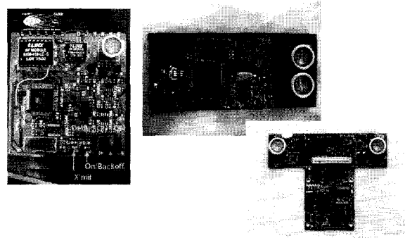
그림 6 크리켓 장치
