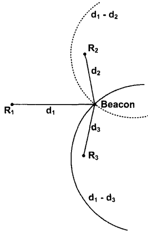
그림 3 TDoA 방식
