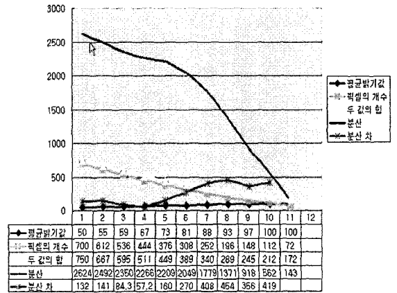
〈그림 8〉 분산과 분산차의 그래프
