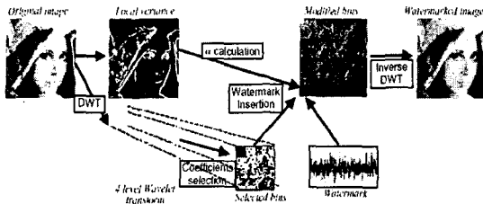
그림 3. 디지털 영상의 임베딩 된 워터마크 순서도. Fig 3. A functional scheme of the view method for embedding a watermark in a digital image
