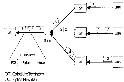
그림 2. 상향전송의 예 (Fig 2. An example of up-stream transmission)
