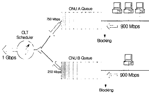
그림 7. 제안된 EPON 대역할당방법 (Fig 7. Bandwidth allocation mechanism of proposed scheme)
