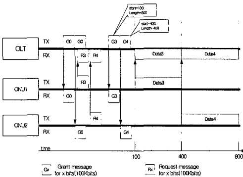
그림 5. MPCP에 의한 상향채널의 대역할당 절차 (Fig 5. Bandwidth allocation step of up-stream channel with MPCP)
