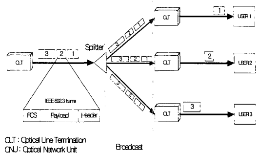
그림 1. 하향전송의 예 (Fig 1. An example of down-stream transmission)
