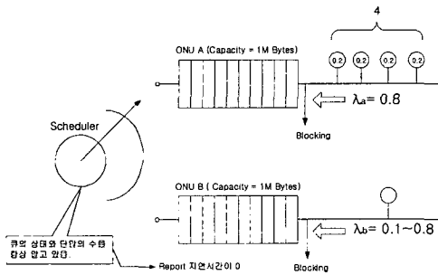
그림 10. 시뮬레이션 모델 (Fig 10. Simulation model)
