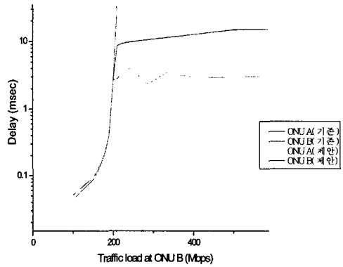
그림 15. 시스템 지연시간 비교 (Fig 15. comparison of system time)
