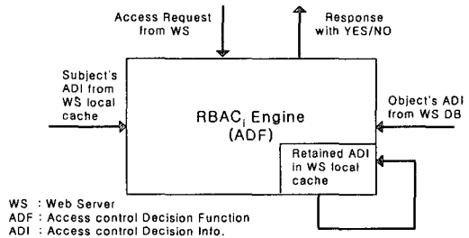
그림 5. RBAC 엔진의 접근 제어 결정 Figure 5. Decision of Access Control by RBAC Engine
