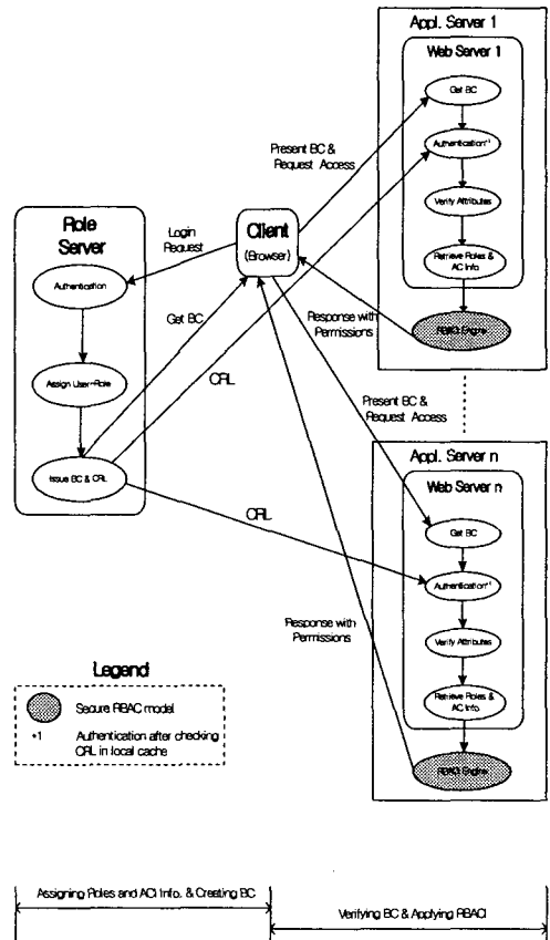
그림 4. SRBAC의 웹상에서의 동작 메커니즘 Figure 4. Operating Mechanism of SRBAC on WWW
