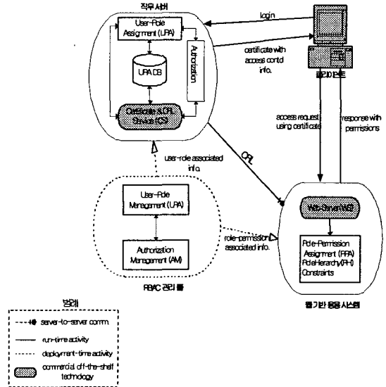
그림 1. 유저-폴 방식의 시스템 아키텍처 Figure 1. System Architecture using UPM
