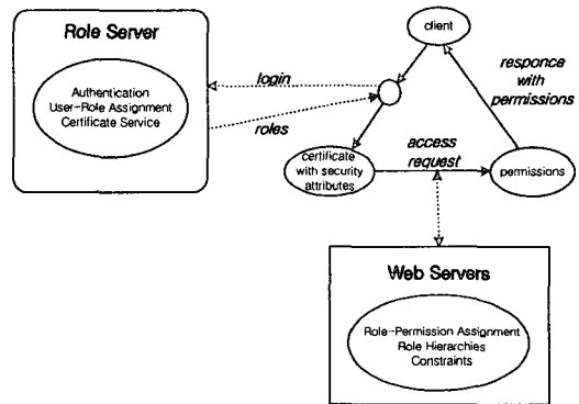
그림 2. 안전한 직무 정보 전달 매커니즘 Figure 2. Secure Mechanism for Role Information Transfer
