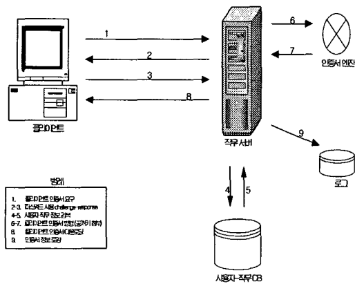
그림 3. 번들 인증서 발행 절차 Figure 3. Procedure of Issuing Bundled Certificates
