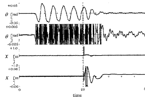
(d) l = 8 m, m_L = 42.2 ton
