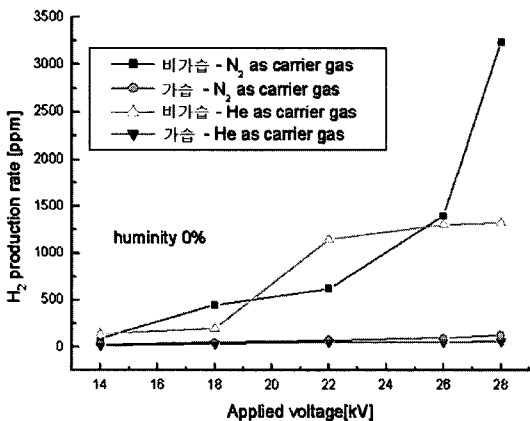
그림 6. 가습의 영향.
