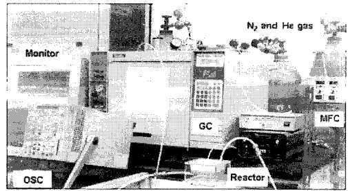
그림 1. 실험장치 구성.
