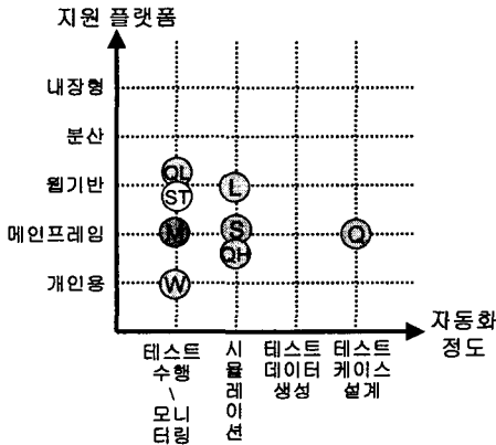
그림 5. 테스트 도구의 분석(지원 플랫폼-자동화 정도) Fig. 5 Analysis of Testing Tools (Supporting Platform-Automatic Level)
