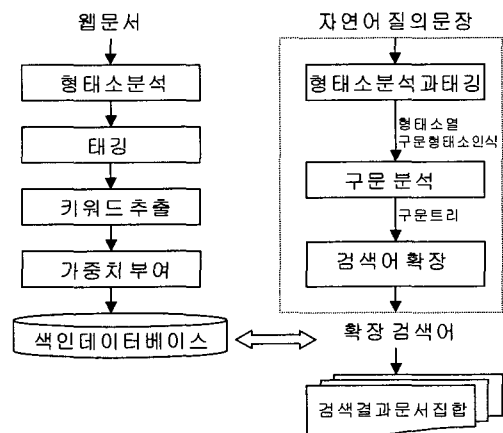
그림 1. 자연어 검색부와 색인부
