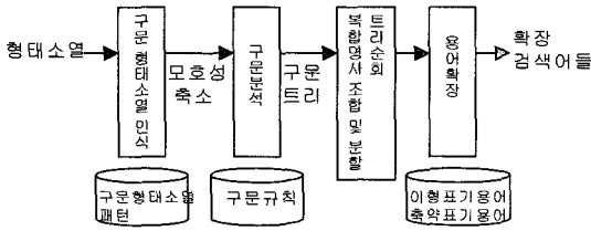
그림 4. 질의문 분석과 검색어 확장
