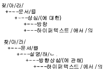
그림 2. 구문분석과 트리
