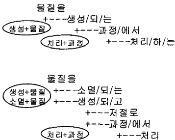
그림 3. 구문트리와 복합명사
