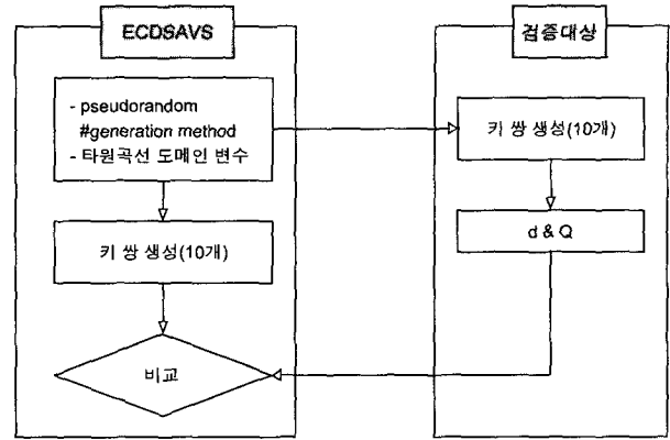
(그림 2) 키 쌍 생성
