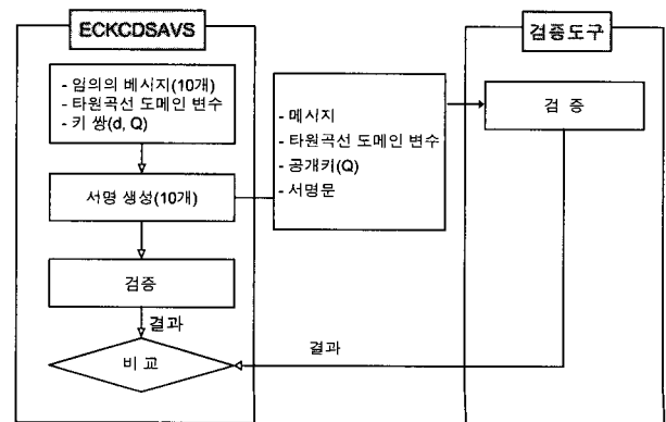
(그림 9) 전자서명 검증
