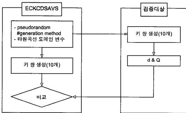
(그림 7) 키 쌍 생성
