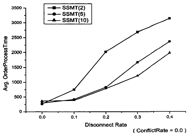
(그림 13) DisconnectRate 변화에 따른 SSMT간 평균주문처리시간
