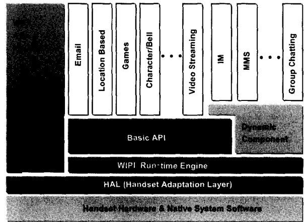
(그림 1) WIPI 플랫폼 개념적 구조도
