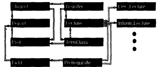
(그림 4) Database E-R Diagram
