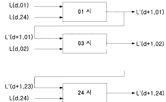
그림 6. Series-parallel 예측 모델. Fig. 6. Series-parallel prediction model.
