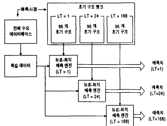
그림 2. 제안된 단기 전력 수요 예측 시스템. Fig. 2. The propose short term electrical load forecasting system.
