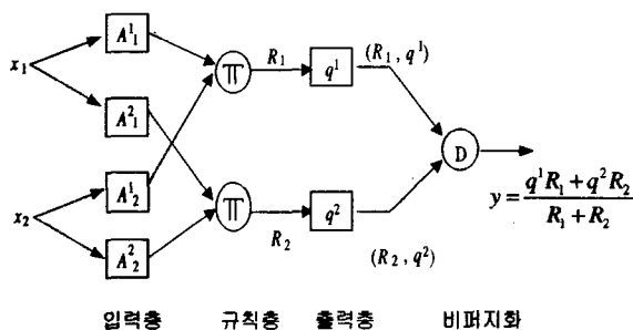
그림 1. 뉴로-퍼지 시스템의 구조. Fig. 1. Architecture of a neuro-fuzzy system.
