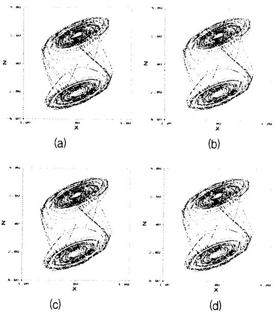
그림 5. 각단의 위상 공간 Fig. 5 Phase portrait of each stage
