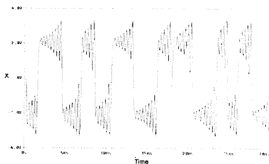
(d) v_{c4} 단의 시계열 데이터 (d) Time series of v_{c4}
