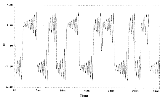
(b) v_{c2} 단의 시계열 데이터 (b) Time series of v_{c2}
