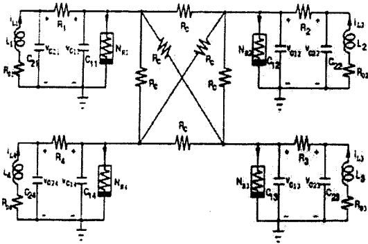
그림 3. Chua's 회로를 이용하여 구성된 Small World 네트워크
