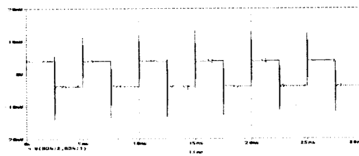
그림 9. 복원 신호 Fig. 9 Recover signal
