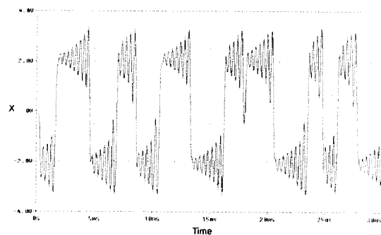
(a) v_{c1} 단의 시계열 데이터 (a) Time series of v_{c1}
