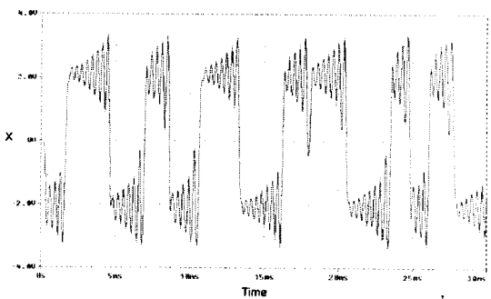
(c) v_{c3} 단의 시계열 데이터 (c) Time series of v_{c3}
