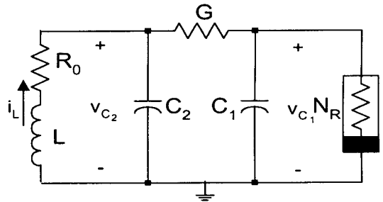
그림 2. Chua's 회로 Fig. 2 Chua's circuit
