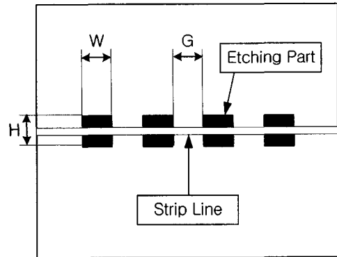
그림 3. 셀의 크기와 간격에 따른 모양의 변화를 보여줄 기본 모양
