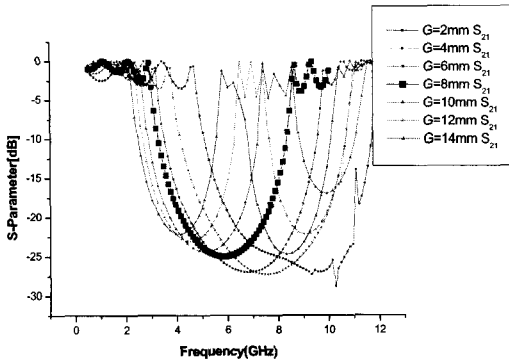
그림 4. G를 변화시켜 가면서 본 주파수특성 (Simulation)
