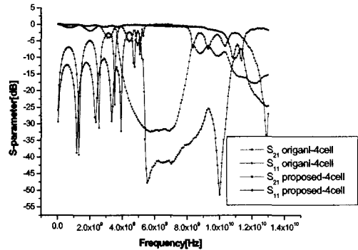
그림 8. 초기에 제작된 적은 반사 손실을 갖는 PBG 구조와 주파수특성
