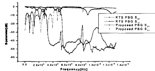
그림 9. 초기에 제작된 광대역 저지특성을 갖는 PBG 구조와 주파수특성
