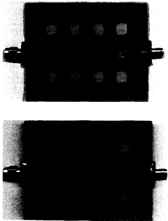
(a) 기본적인 PBG 구조의 앞면과 뒷면 (a) Top and Bottom of fundamental PBG Structure
