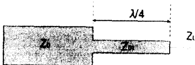
그림 4. λ/4 변환기
