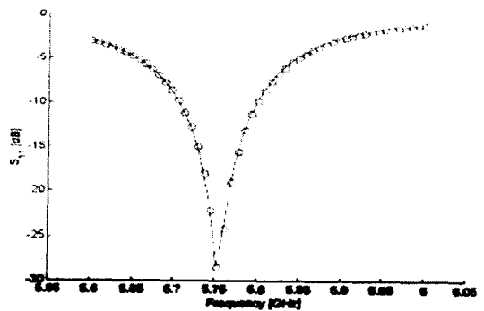
그림 6. 설계된 안테나의 주파수에 따른 S 11
