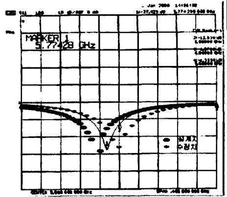
그림 11. 제작된 안테나의 S_{11}
