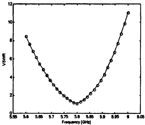
그림 9. 수정된 안테나의 VSWR
