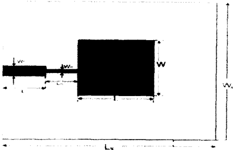
그림 3. 구형 마이크로스트립 안테나 구조
