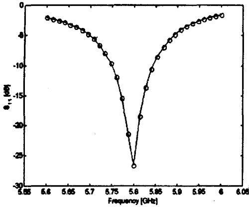
그림 8. 수정된 안테나의 주파수에 따른 S_{11}
