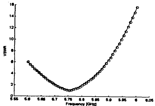
그림 7. 설계된 안테나의 VSWR
