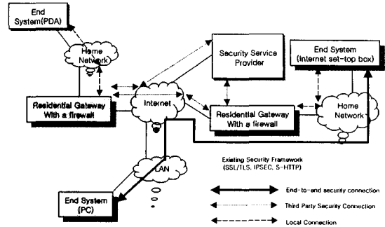
그림 2. 홈 네트워크 보안기술 구성도 Fig 2. Configuration of Security Flow for Home Network
