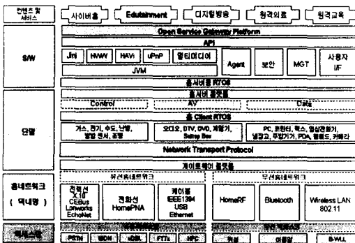
그림 1. 홈 네트워크의 미들웨어의 구성도
