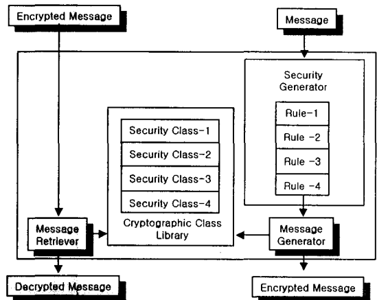
그림 3. 적응형 종단간 홈 네트워크 보안 프레임 Fig 3. Adaptive End-to-End Home Network Security Framework
