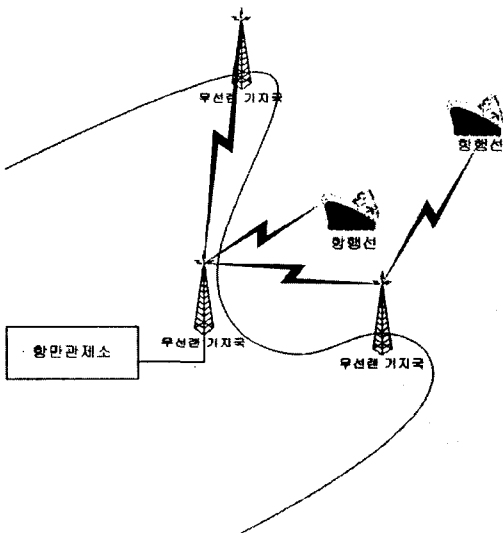
그림 3-1. 무선랜을 이용한 항만통신망
