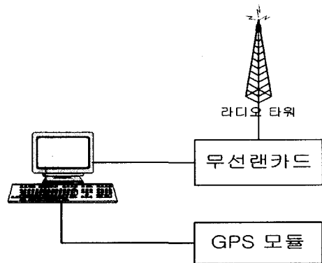
그림 3-3. 사용자 시스템의 구성도
