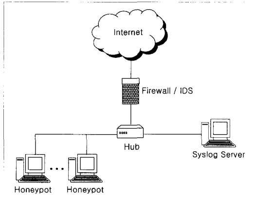
[그림 2] 허니넷 시스템
