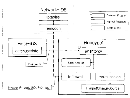
[그림 13] 텔넷 세션 이동 과정
