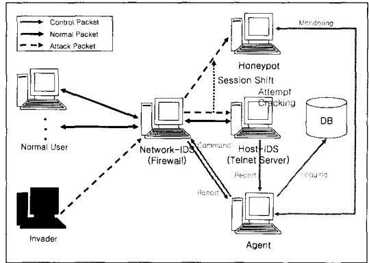
[그림 12] 시나리오 C의 동작 개념도
