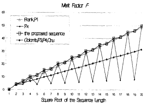
그림 1. \sqrt{N} 에 대한 Merit Factor F
