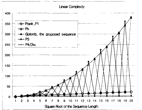
그림 4. \sqrt{N} 에 대한 선형 복잡도
