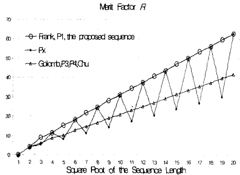
그림 2. \sqrt{N} 에 대한 Merit Factor R
