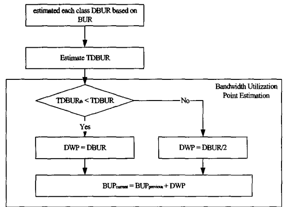
그림 2. 각 클래스별 BUP 값 산출 순서도 Fig. 2. Each class BUP measurement flowchart
