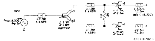
(a) 회로도
