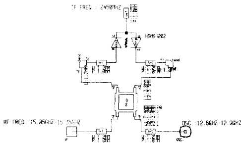
(a) 회로도
