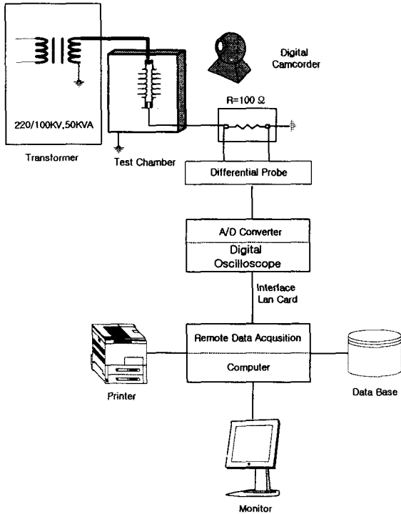
그림 1 전체 시스템 구성도 Fig. 1. Whole system diagram
