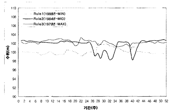
그림 7. 춘천댐 운영곡선(수위)
