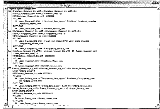
그림 5. 북한강 유역 모형의 방정식 레벨
