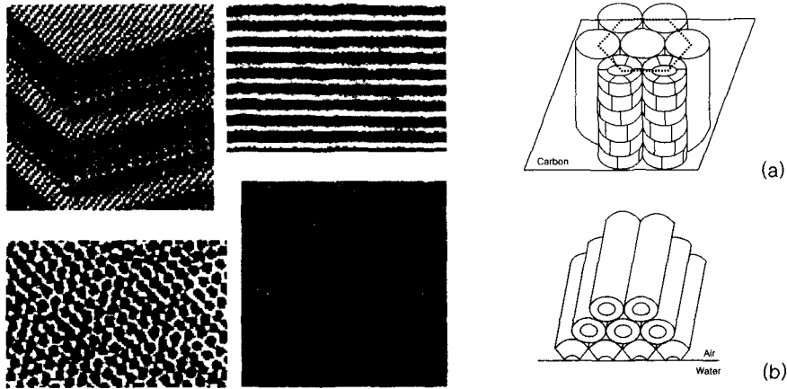
그림 6. Column 형태의 초분자 구조체의 전자현미경 사진과 표면조절에 의한 column 배향 메카니즘 모식도: Homeotropic column 배향조절은 hydrophobic 표면에서, planar 구조는 polar 표면에서 주로 형성된다.
