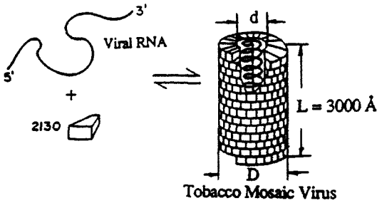
그림 2. Tobacco Mosaic Virus의 자기조립 메커니즘.
