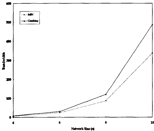
<그림 10> 지역 참조성이 0.8일때 네트워크 크기에 따른 BW
