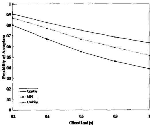
<그림 11> 1024×1024 Combine MIN에서 부하 변화에 따른 PA
