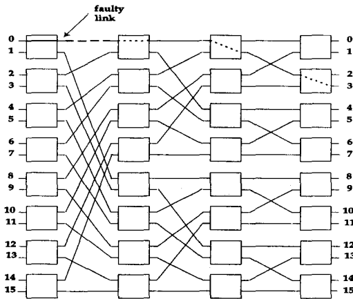
<그림 5> 16x16 MIN에서 링크 오류 발생시 대체 경로의 부재
