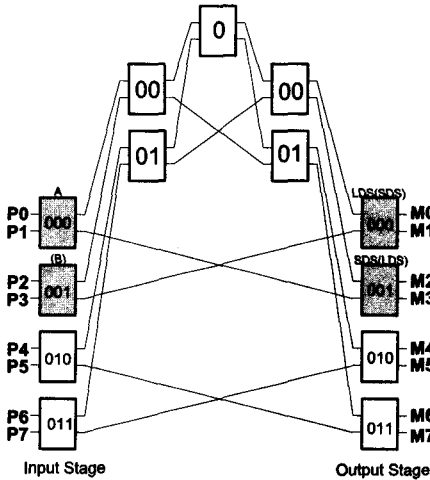
<그림 2> Combine MIN에서의 LDS와 SDS
