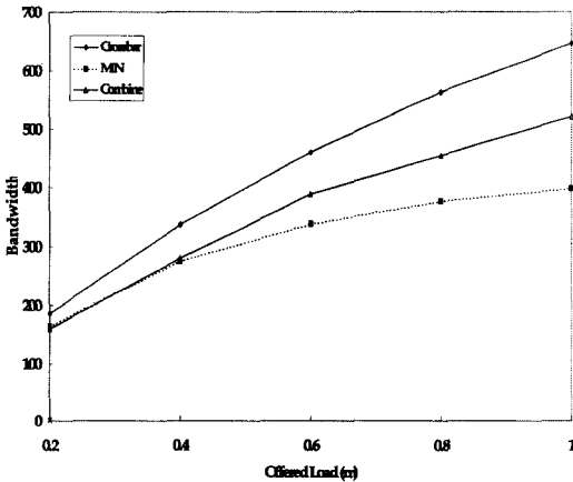
<그림 8> 네트워크의 부하 변화에 따른 BW
