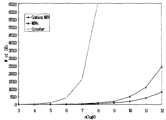
<그림 7> 시스템 크기에 따른 사용되어지는 스위칭 소자의 수
