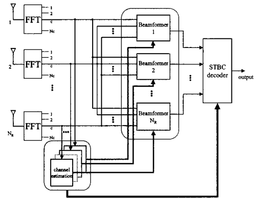
그림 4. 빔형성기의 구조
