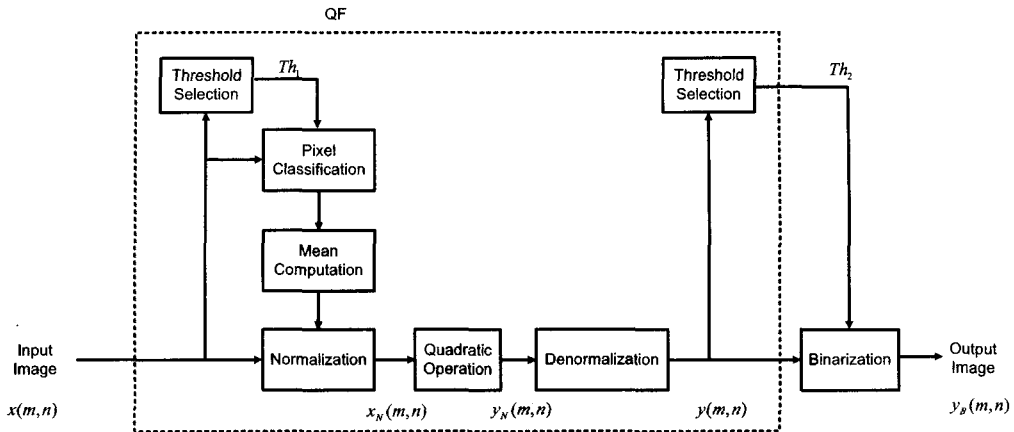
그림 1. 기존의 QF를 이용한 전역 이진화의 블록도 Fig. 1. Block diagram of a conventional GB using QF.
