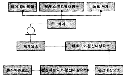
(그림 6) 체계분산환경기술서(SV-6) CADM
