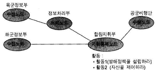
(그림 7) 운용노드연결기술서(OV-2) 예
