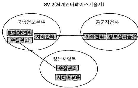
(그림 9) 체계인터페이스기술서 아키텍처 산출물
