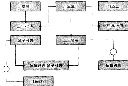
(그림 4) 운용노드연결기술서(OV-2) CADM
