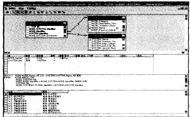
(그림 10) 노드와 체계 관련 질의 및 결과
