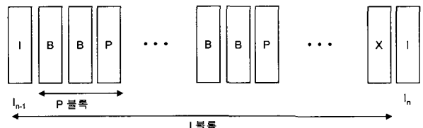
(그림 4.3) I 블록 내부의 P블록 및 B픽처 구조
