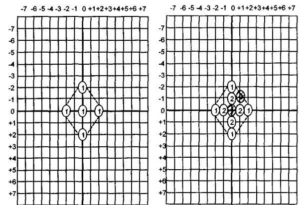
(a) 초기탐색점 배치
