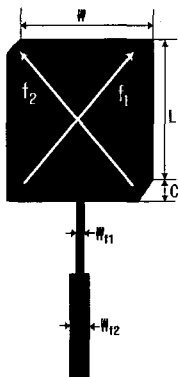
그림 3. 원편파 발생을 위해 코너 절단 방식을 채택한 초전도 안테나의 단일소자 패턴.
