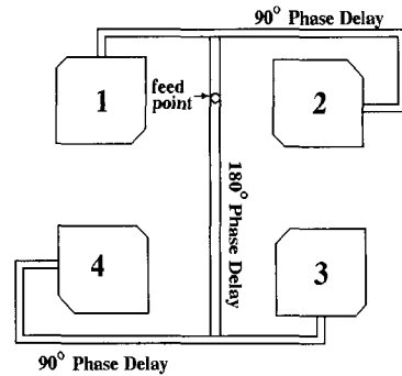
그림 4. 원편파 배열 안테나를 위한 순차적 순환 급전방식의 개략도.
