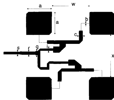
그림 5. 원편파 발생을 위해서 순차적 순환 급전방식을 이용한 4소자 배열의 구조.
