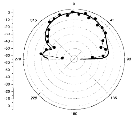
그림 8. 제작된 초전도 배열 안테나의 \phi=90^\circ 평면 방사패턴.
