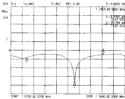
그림 9. 77 K에서 초전도 안테나의 반사손실. Fig. 9. Return loss for our HTS antenna array at 77 K.
