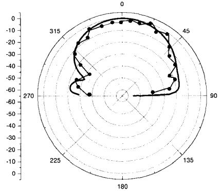
그림 7. 제작된 초전도 배열 안테나의 \phi=0^\circ 평면 방사패턴.
