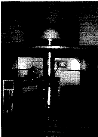
그림 6. 안테나 측정을 위한 냉각기 사진. Fig. 6. Photograph of cryostat for antenna measurement.
