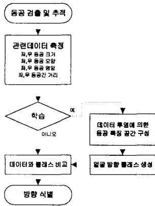
그림 8. 얼굴 방향 식별 알고리즘 순서도
