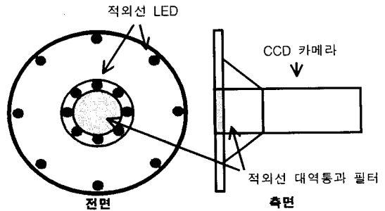
그림 1. 하드웨어 구성: 능동적 적외선 조명 카메라 Fig 1. Hardware setup: the camera with an active IR illuminator.
