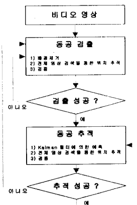
그림 2. 동공 탐지 및 추적 시스템 순서도
