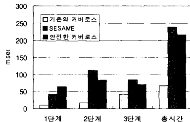
그림 8. 티켓 발행 시간 측정 그래프(다중 영역) Fig. 8. Determination graph of ticket issuing time(multi-area)
