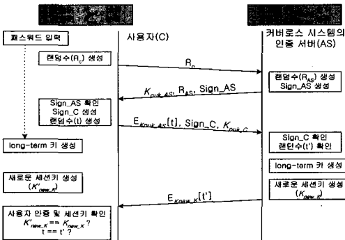
그림 6. 안전한 인증 프로토콜 Fig. 2. Secure-authentication protocol
