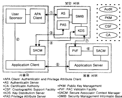
그림 1. SESAME 시스템의 구조 Fig. 1. Structure of SESAME system
