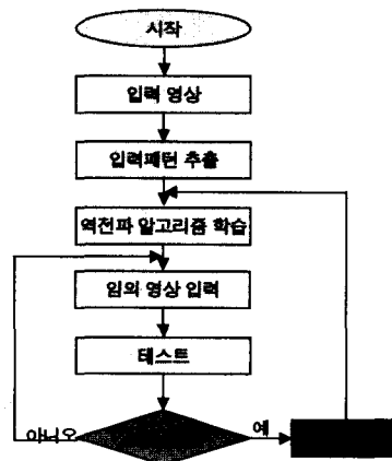
그림 9. 학습 알고리즘
