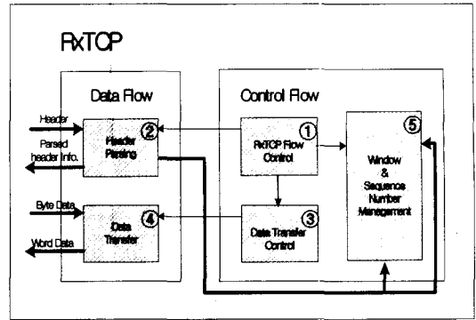
그림 5. Rx TCP 블록 다이어그램
