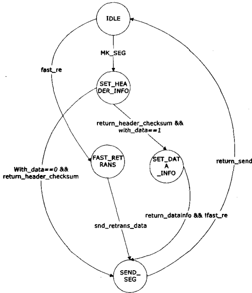
그림 11. Tx TCP FSM
