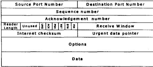
그림 1. TCP 헤더 구조
