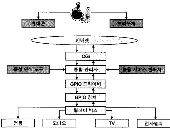
(그림 6) 사용자 요청의 전체적인 제어 흐름
