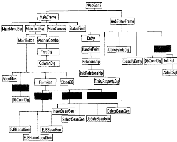
(그림 8) WebSiteGen2의 컴포넌트 계층구조
