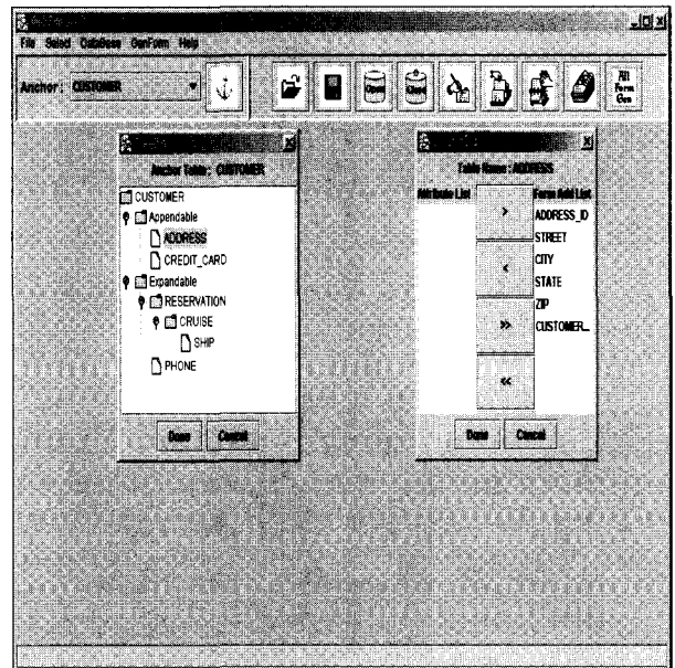
(그림 4) TreeDlg와 ColumnDlg 다이얼로그 박스
