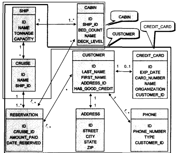
(그림 6) 각 품이 커버하는 개체 그룹
