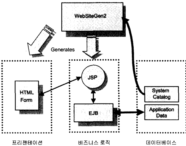
(b) 기존 데이터베이스로부터 응용 생성
