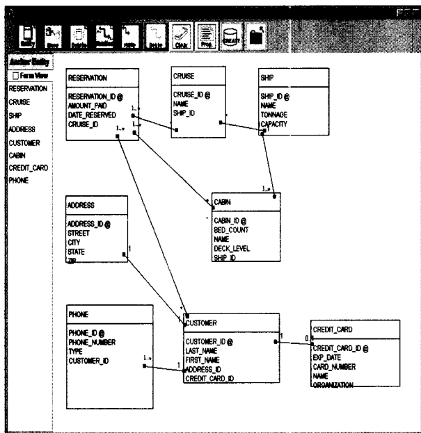
(그림 1) Titan 응용의 클래스 다이어그램
