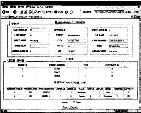
(그림 5) Titan 응용의 Update/Delete CUSTOMER 품
