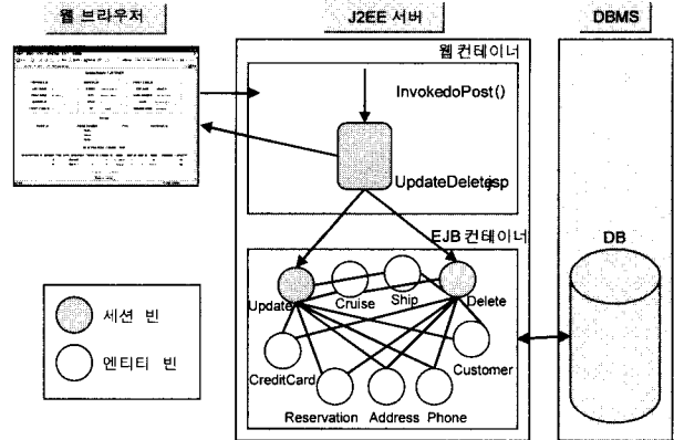
(그림 7) Titan 응용의 구조
