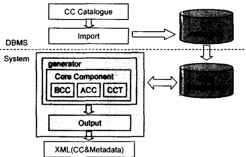
(그림 5) 핵심 컴포넌트 저장을 위한 시스템 구성도
