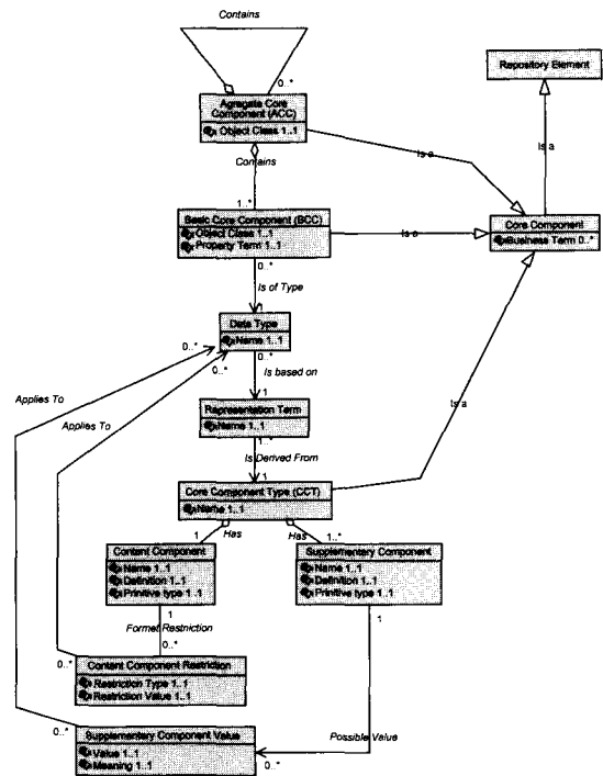
(그림 4) 핵심 컴포넌트의 유형과 저장을 위한 UML 모델
