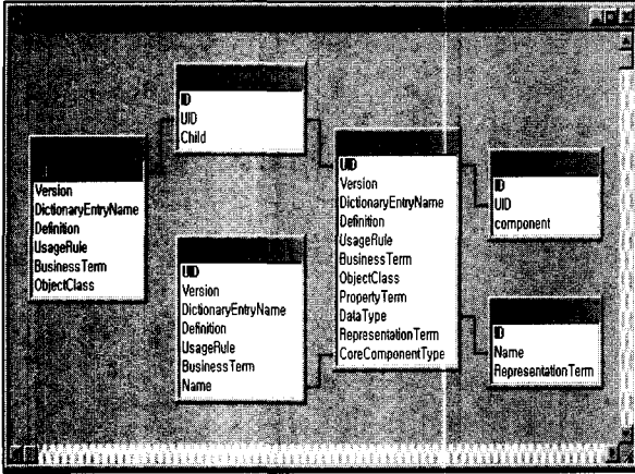
(그림 11) 테이블 관계도
