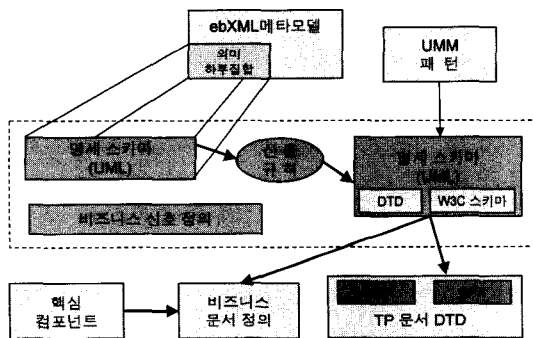
(그림 2) 비즈니스 프로세스 명세 스키마
