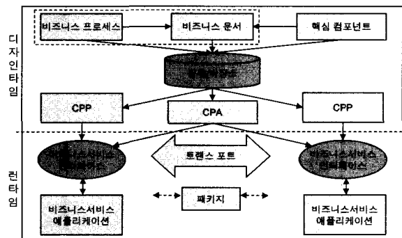
(그림 1) ebXML 구성요소
