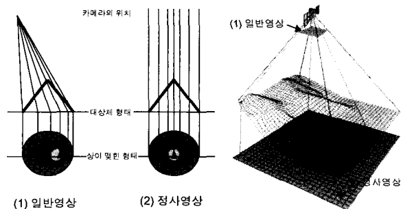
(그림 3) 정사영상의 개념도
