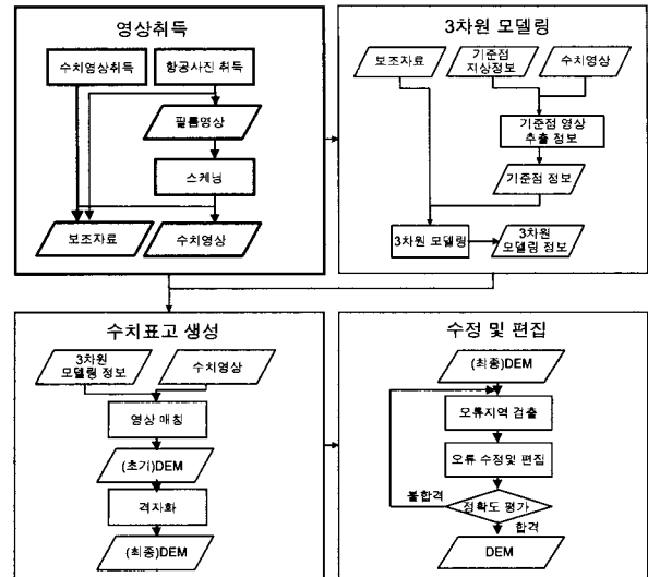
(그림 1) 수치표고모델 제작 절차 개념도
