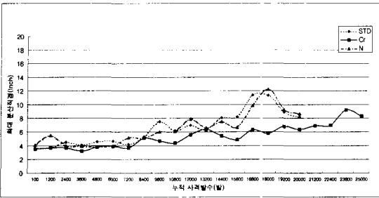
[그림 5] 각 표면처리총열별 분산도 비교
