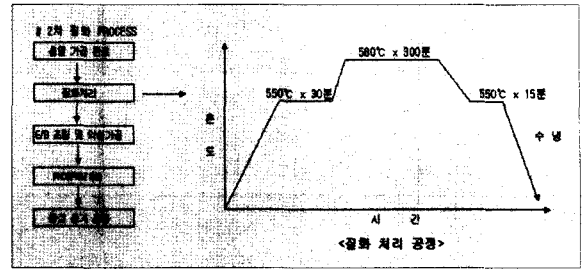
[그림 3] 최적 질화처리 공정
