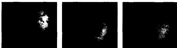
a) 약실부 b) 중앙부 c) 총구부 [그림 11] 질화처리총열 염수분무 내경(5배율)
