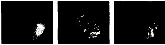
a) 약실부 b) 중앙부 c) 총구부 [그림 9] 표준총열 염수분무 내경(5배율)
