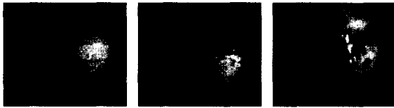
a) 약실부 b) 중앙부 c) 총구부 [그림 10] 크롬도금총열 염수분무 내경(5배율)
