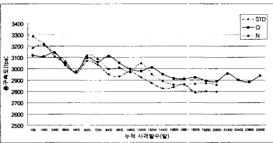
[그림 6] 각 표면처리총열별 총구속도 비교
