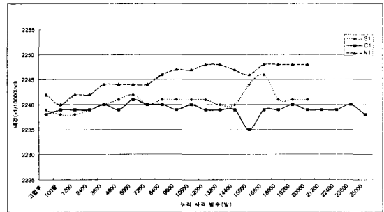
[그림 8] 총구부(1번지점) Groove 치수변화
