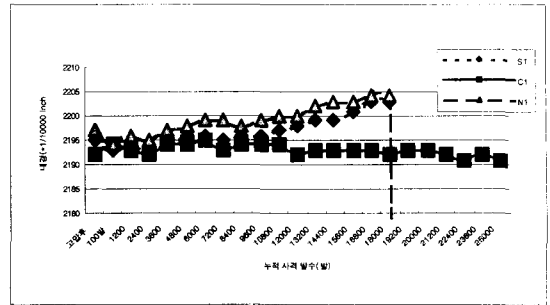
[그림 7] 총구부(1번지점) Land 치수변화
